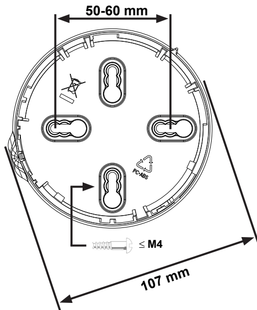
Figura 1: Montaggio B501RF
