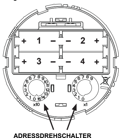
Abbildung 4: Batterieinstallation und Adressdreheshalter
