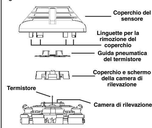
Figura 2: Pulizia del sensore
