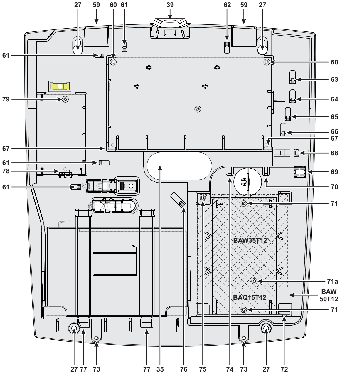
Figura 5 Fijación del contenedor Plástico.
