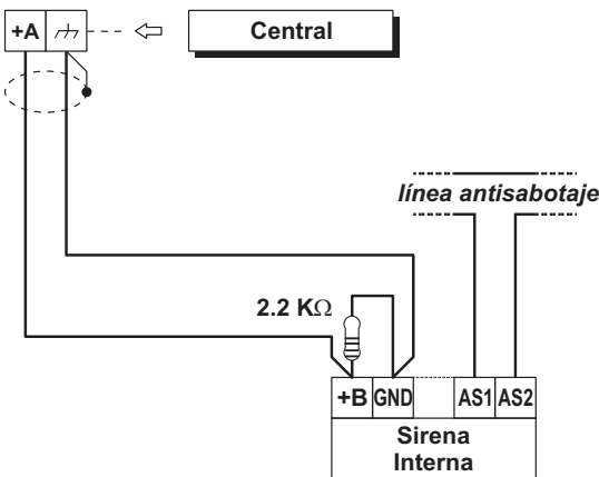
Figura 17 Conexión de una Sirena Interna a una salida Supervisada por la Centrale.
