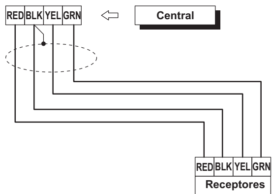
Figura 29 Conexión del Receptor a la Central.
