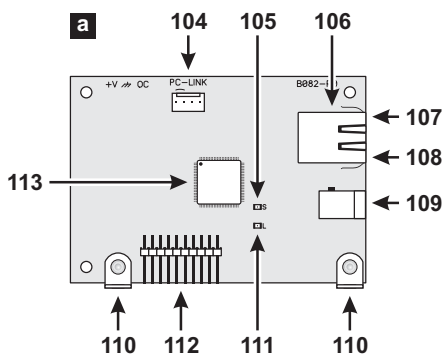
Figura 7 Partes del Módulo IP ABS-IP (a) y de Puente WiFi ABS-VAP11N (b).
