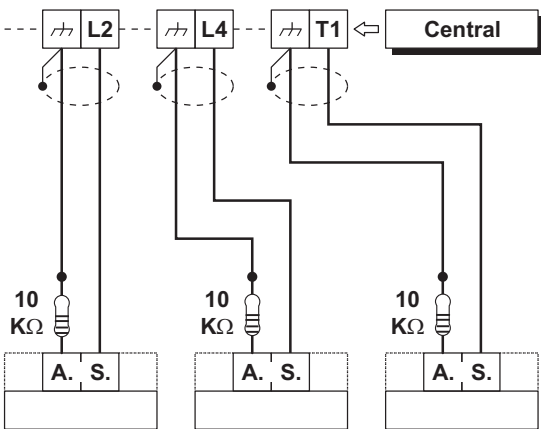
Figura 19 Conexión de tres contactos antisabotaje a tres zonas tipo 24h con SEOL Supervisada, los bornes [A.S.] son el contacto antisabotaje, Normalmente Cerrado, del dispositivo.
