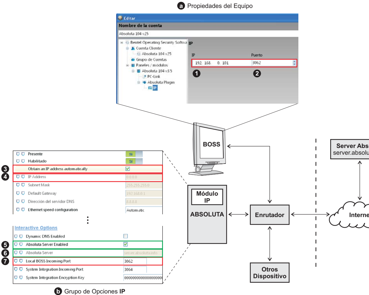
Figura 30 Conexión vía IP.
