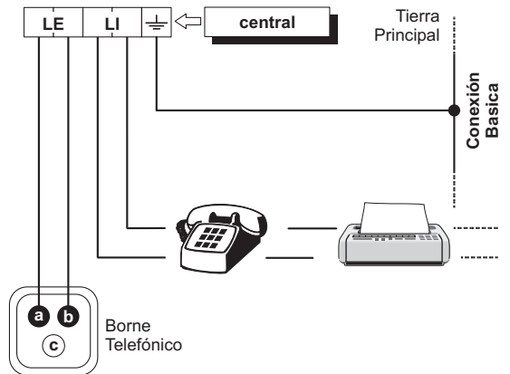
Figura 20 Conexión de la línea telefónica a la Central.
