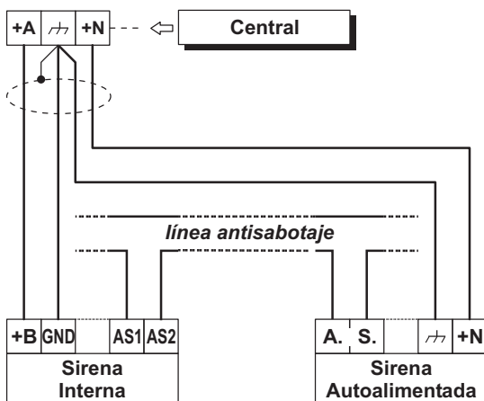
Figura 16 Conexión de una Sirena Autoalimentada y de una Sirena Interna a la Salida n°1 de la Centrale.
