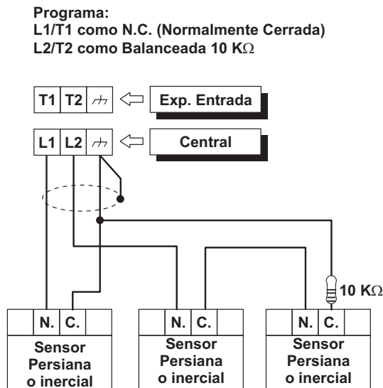
Figura 14 Conexión de sensores Inerciales (sólo para las zonas de la central) y Contactos para Persianas: conexión de un sensor a una zona N.C. de dos sensores a una zona Balanceada 10K.
