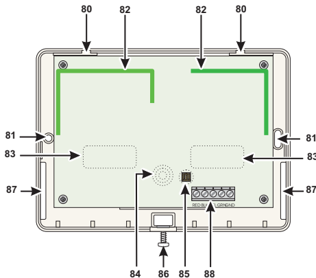
Figura 28 Partes del Receptor.
