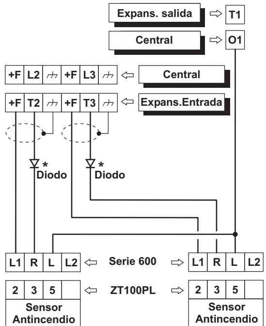
Figura 15 Conexión de 2 sensores antiincendio a zonas con Balance Normalmente Abierto (* Sólo con la serie 600).
