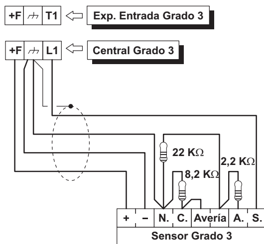
Figura 13 Conexión de un sensor a una Zona con el Conexión Triple End of Line .
