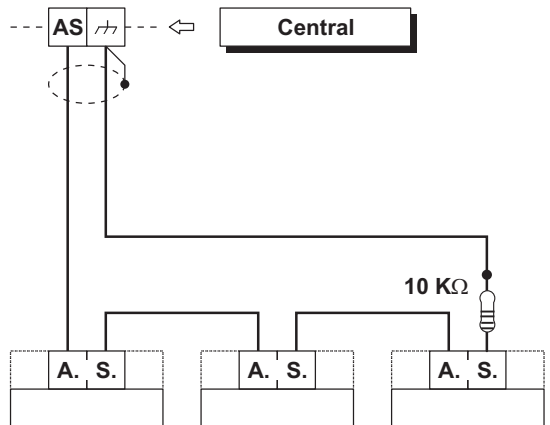
Figura 18 Antisabotaje de la central: Los bornes [A.S.] son el Contacto Antisabotaje, Normalmente cerrado, del Dispositivo.
