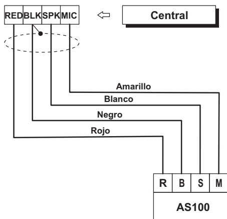
Figura 21 Conexión de l'AS100 a la central.
