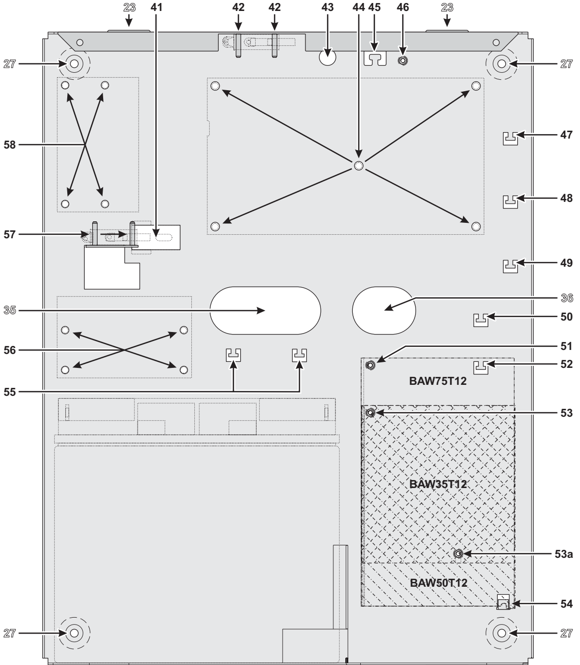
Figura 4 Fijación del contenedor Metálico.
