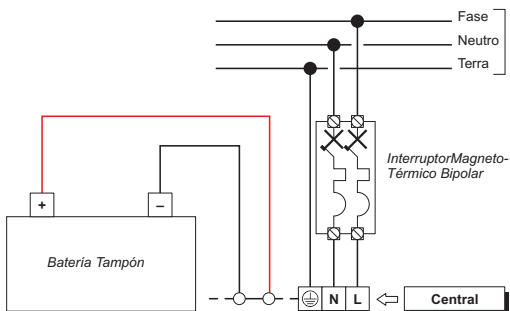
Figura 22 Conexión de la alimentación.
