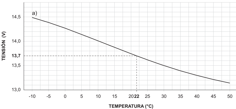
Figura 23 Gráfico para regular la tensión de salida del Alimentador en función de la temperatura de la Sonda Térmica: Identificar en el eje TEMPERATURA (°C) la temperatura de la Sonda Térmica; trazar una línea vertical desde este punto hasta la curva a ; trazar una línea horizontal desde el punto en el cual la línea vertical intercepta la curva a con el eje TENSIÓN (V) ; Regular la tensión de salida del Alimentador en el valor encontrado. Por ejemplo, si la temperatura de la Sonda es de 22 °C, regular la tensión de salida del Alimentador 13,7.
