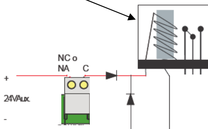
Relé auxiliar para consumos no limitados
