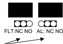
Puentes para configurar relés de avería y alarma como NC o NO
