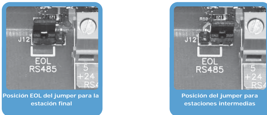
Figura 12 - Posiciones del jumper
