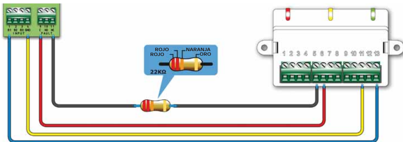
Figura 4 - Diagrama de cableado de una conexión de lazo usando un módulo EM312SR
