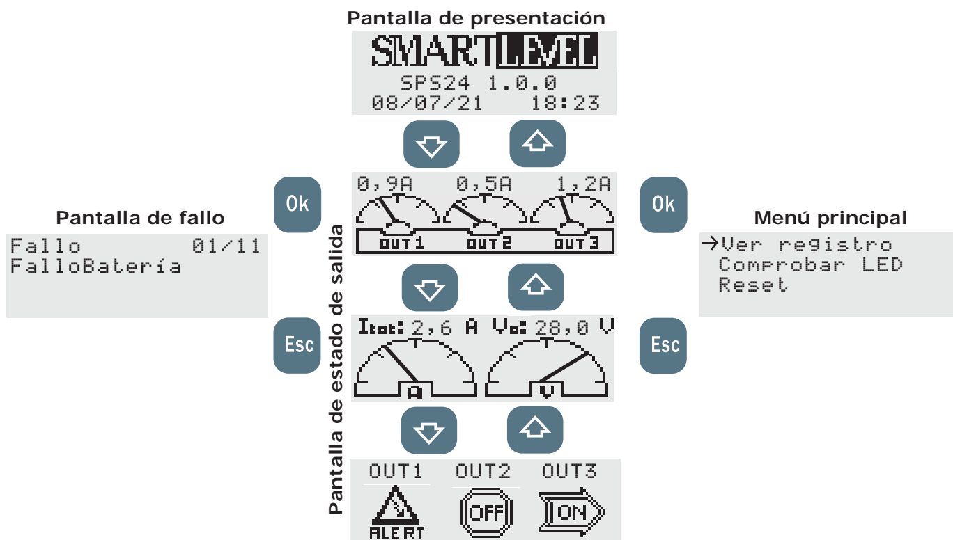
Figura 17 - Navegación en las pantallas del display
