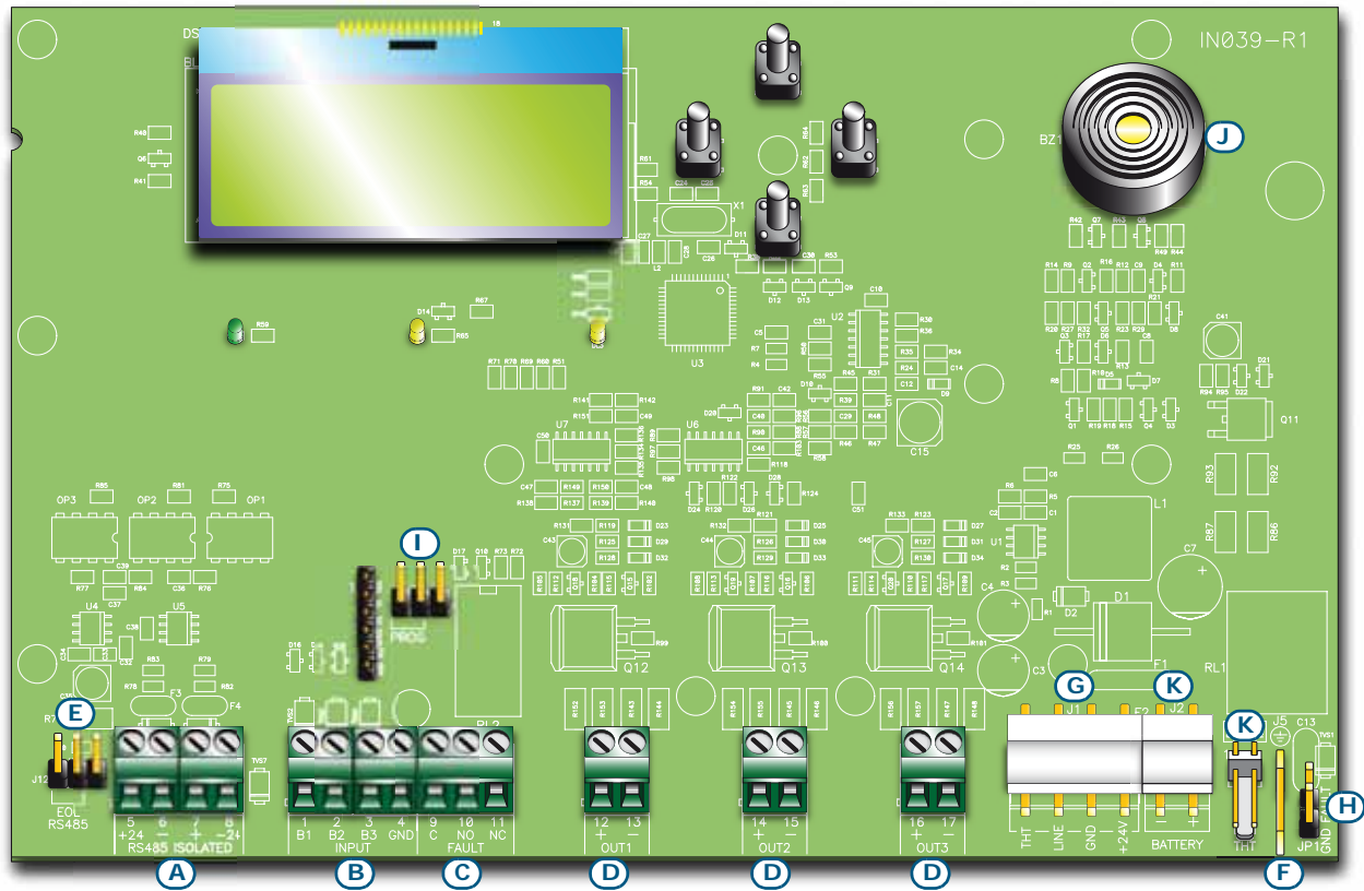
Figura 8 - Placa madre del SmartLevel
