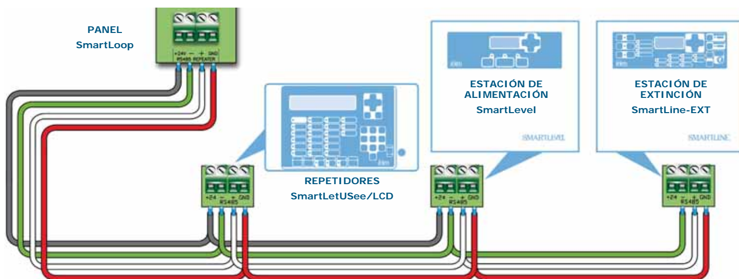
Figura 11 - Conexión BUS RS485
