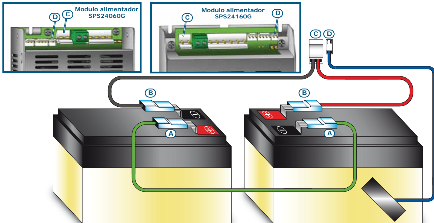
Figura 14 - Conexión de las baterías
