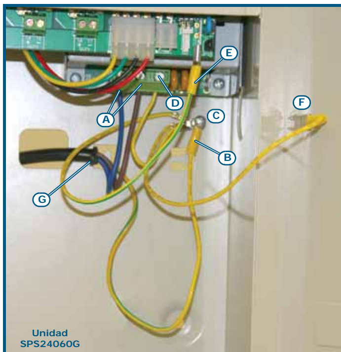
Figura 13 - Conexión de tierra
