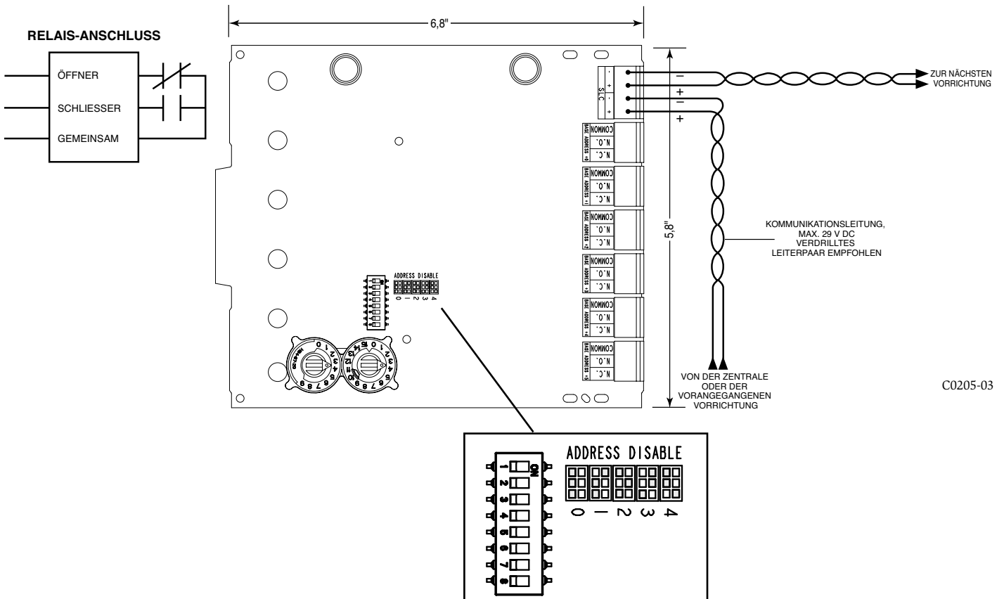
ABBILDUNG 1: VERDRÄHTUNG UND PROGRAMMIERUNG DES NFXI-RM6-MODULS
