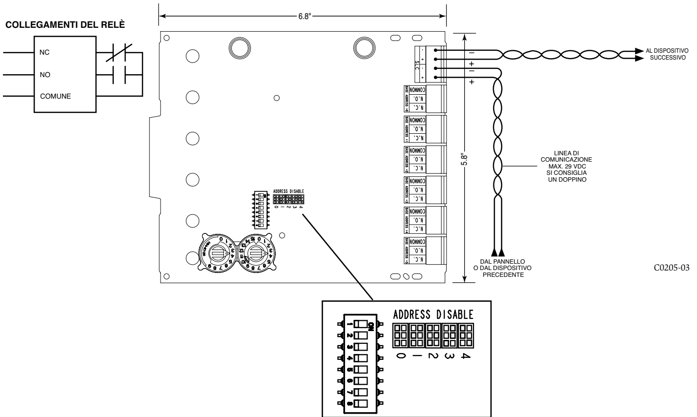
FIGURA 1: CABLAGGIO E PROGRAMMAZIONE DEL MODULO NFXI-RM6
