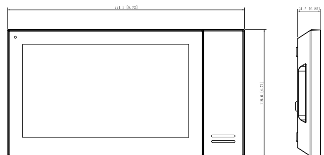
DHI-VTH2421FW-P
