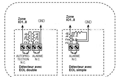
Schéma 2.1 - Exemple de connexion d'un détecteur
