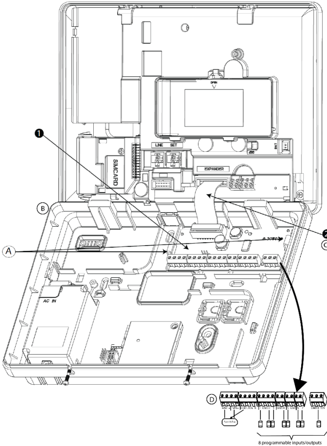
Figura 2.1 - Montaggio e cablaggio del modulo Expander ioXpander-8
