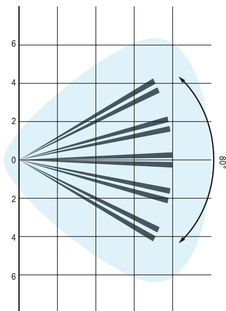
Air2-XIRP200W - vista desde arriba
