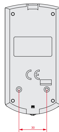
Air2-XDTP200W, Air2-XIRP200W - parte posterior
