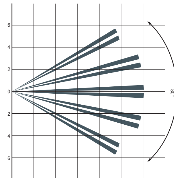
Air2-XIRP200W - vista desde arriba
