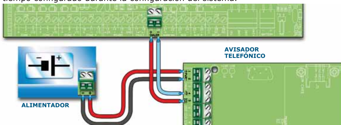
Figura 21 - Conexión de un comunicador telefónico
