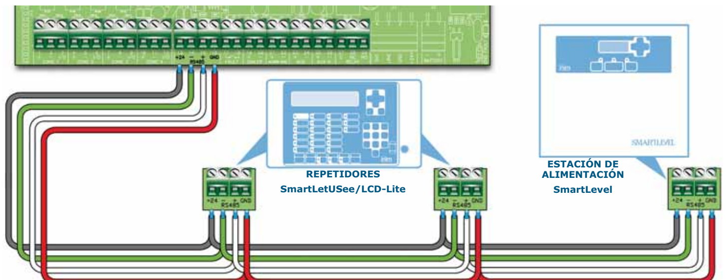
Figura 24 - Conexión BUS RS485
