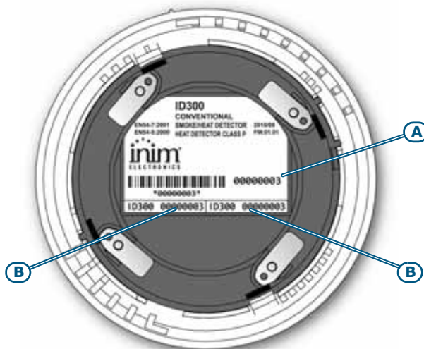
Figura 36 - Parte trasera del detector Iris
