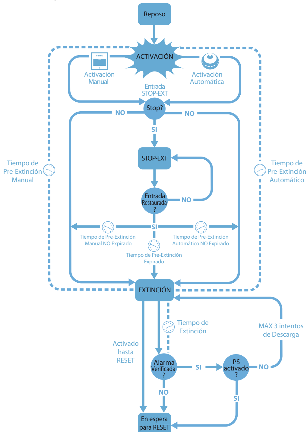
Figura 35 - Módulo de extinción: diagrama de funcionamiento
