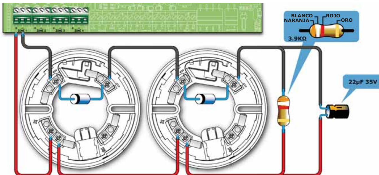
Figura 15 - Conexión de los detectores para la detección también en caso de ausentes
