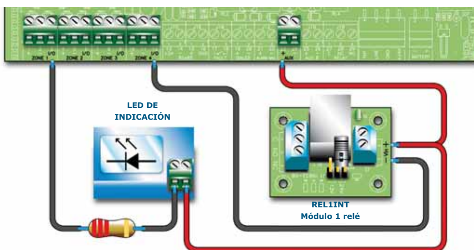
Figura 18 - Conexión de la línea E/S como salida
