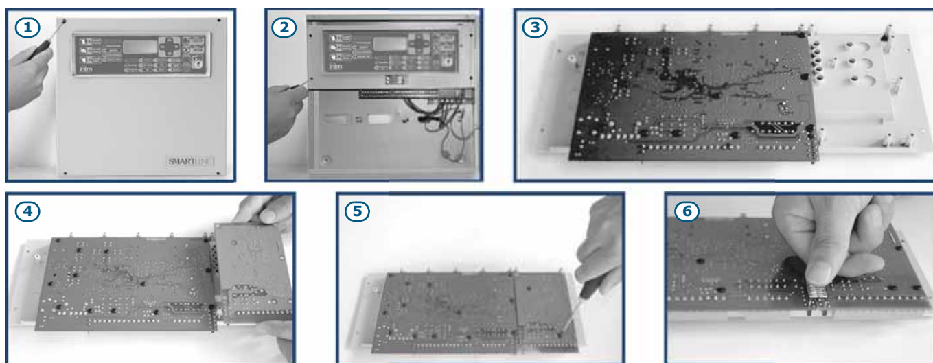
Figura 12 - Montaje del módulo de extinción
