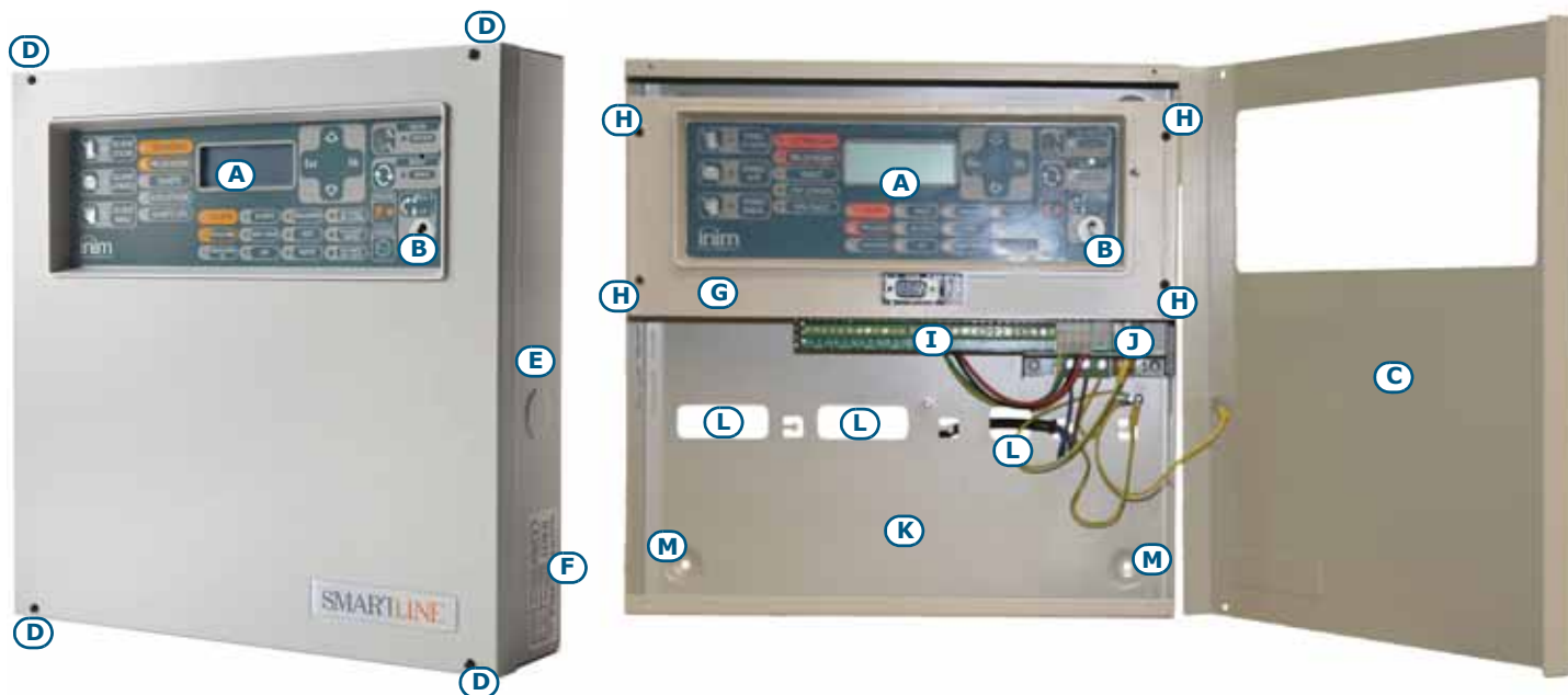
Figura 3 - Exterior y interior de SmartLine020
