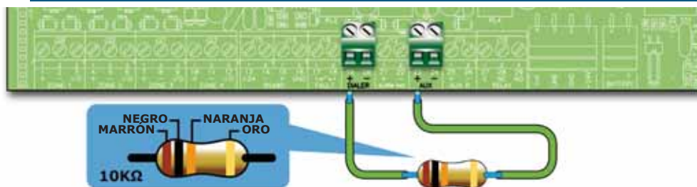
Figura 22 - Conexión salida + DIALER sin comunicador telefónico
