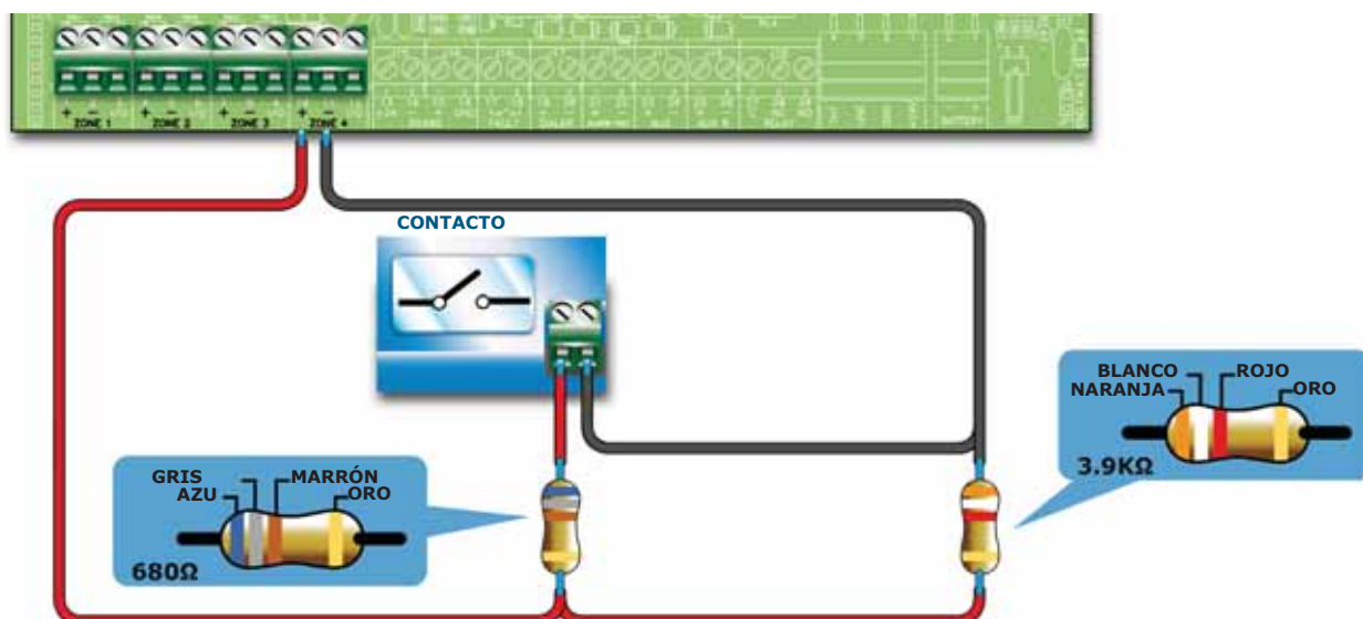
Figura 17 - Conexión a la línea de un contacto genérico
