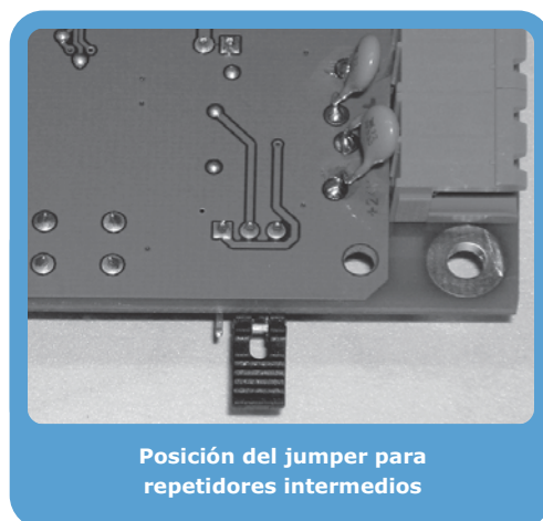
Figura 25 - Módulo SmartLetUSee/LCD-Lite - posición del jumper
