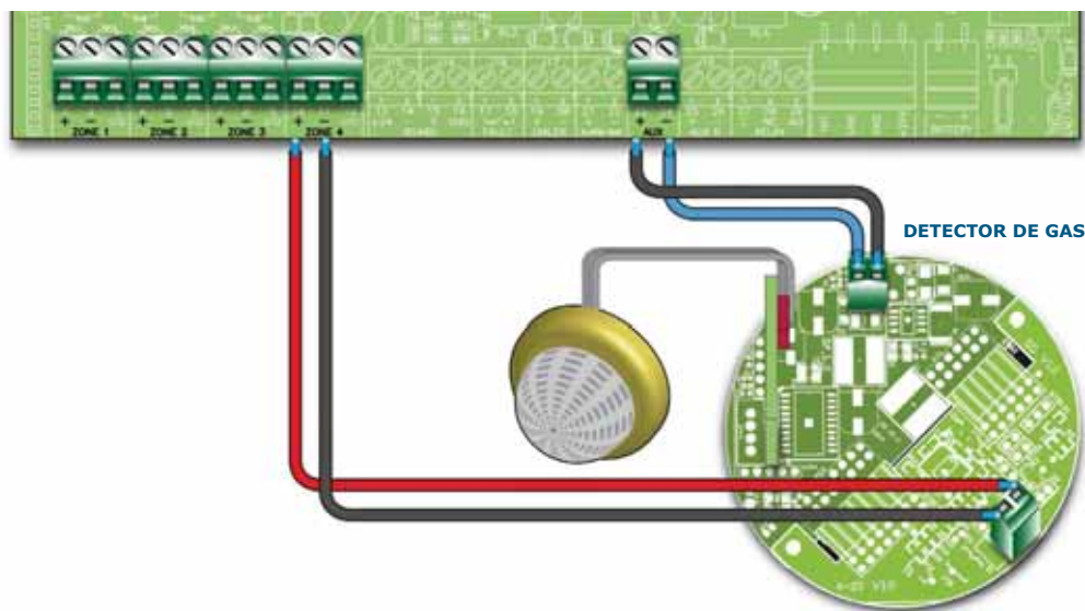
Figura 16 - Conexión de los detectores de gas en la línea de detección
