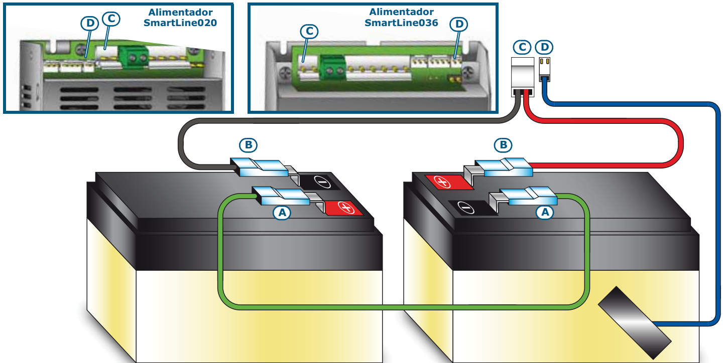
Figura 33 - Conexión de las baterías
