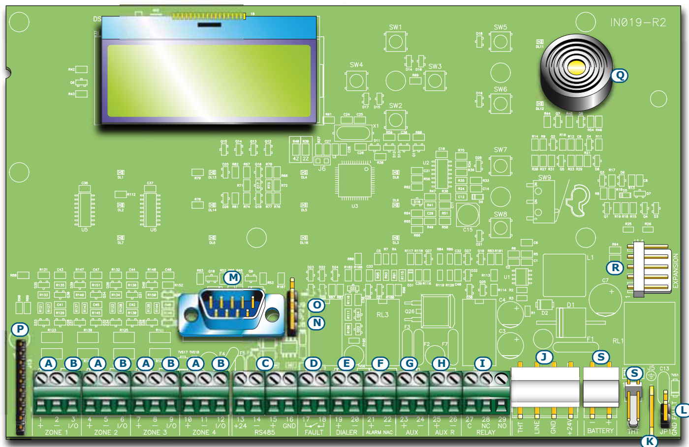
Figura 5 - Módulo SmartLine
