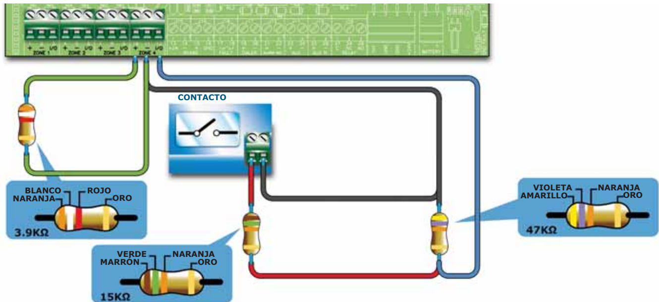
Figura 19 - Conexión de la línea E/S como entrada
