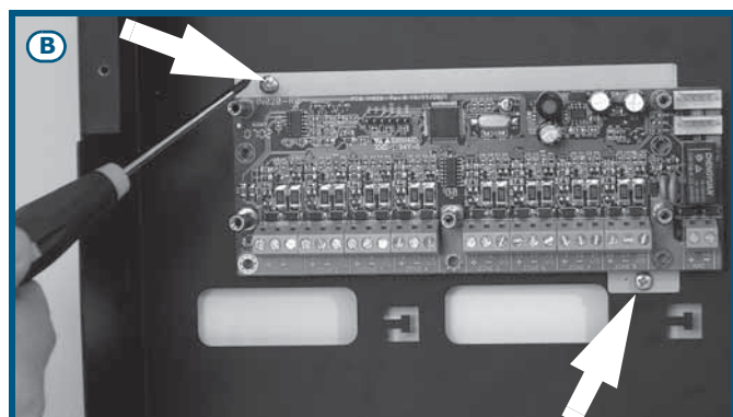
Figura 10 - Montaje del módulo de expansión - 1
