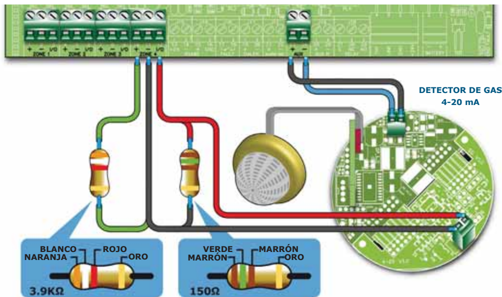
Figura 20 - Conexión de los detectores de GAS 4-20mA
