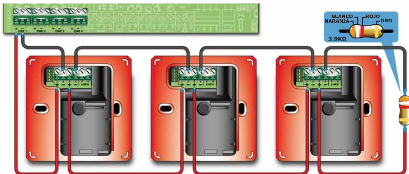
Figura 14 - Conexión de los pulsadores de alarma Iris
