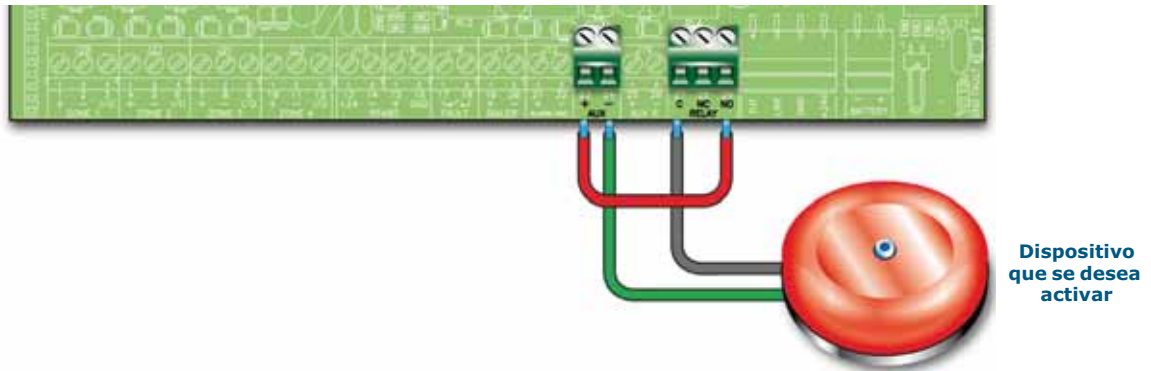
Figura 30 - Conexión de la salida RELAY
