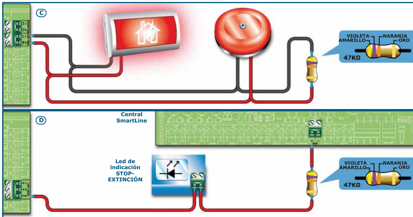
Figura 31 - Módulo de extinción
