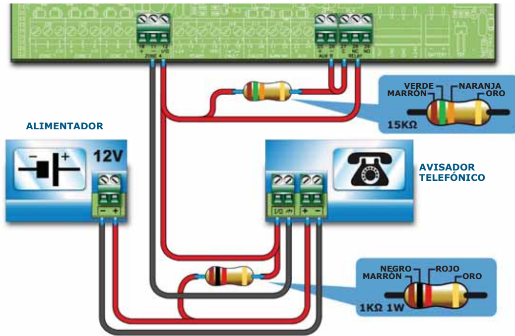
Figura 23 - Conexión de un comunicador telefónico
