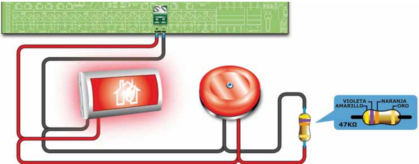
Figura 28 - Conexión de la salida de indicación de alarma
