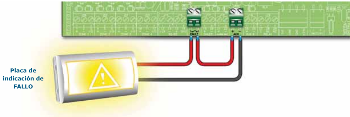
Figura 27 - Conexión de la salida de indicación de la avería
