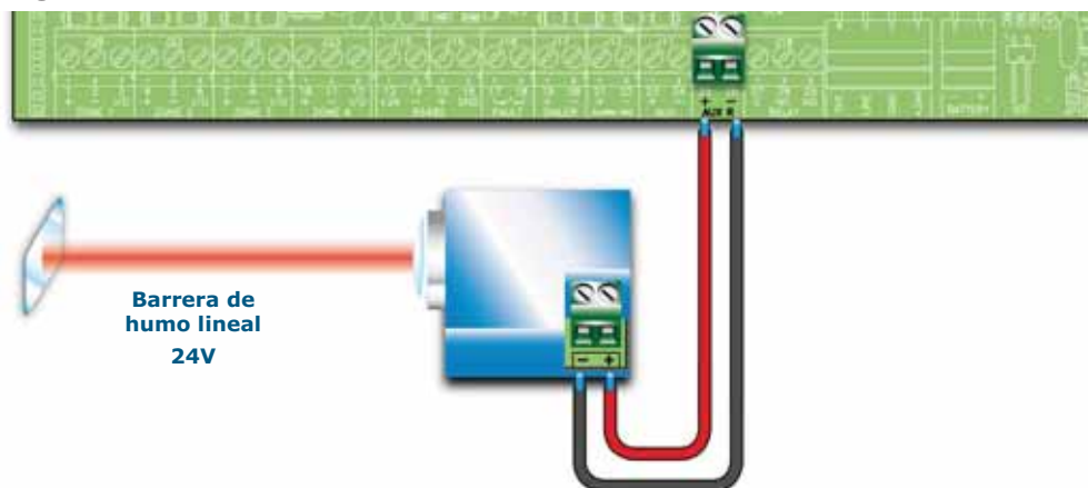
Figura 29 - Conexión de la salida AUX-R
