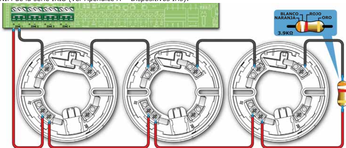
Figura 13 - Conexión de los detectores Iris
