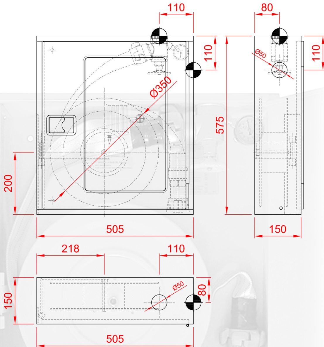
DIMENSIONES EMPOTRAMIENTO
