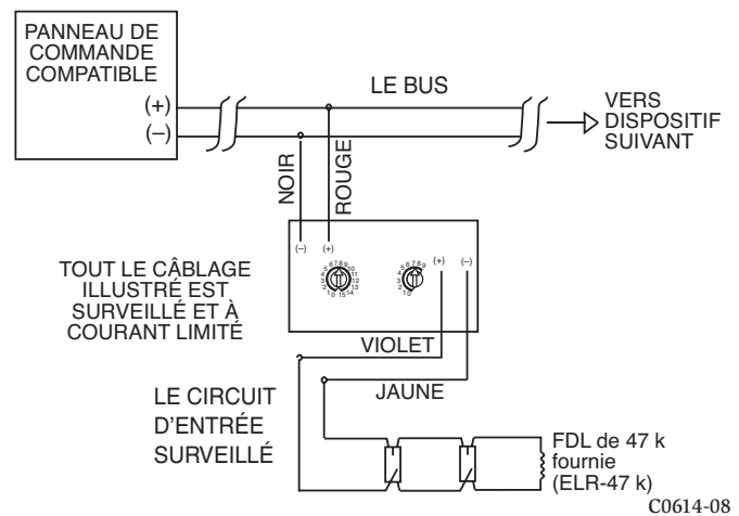
FIGURE 2. CONFIGURATION TYPE D'UN CIRCUIT :
