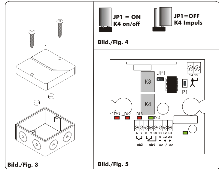
Bild./Fig. 3
