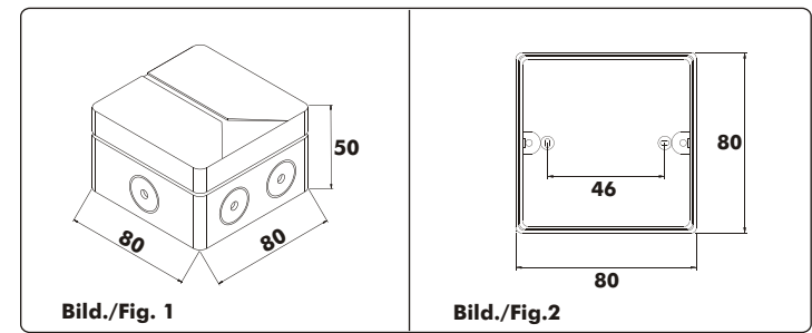
Bild./Fig. 1
