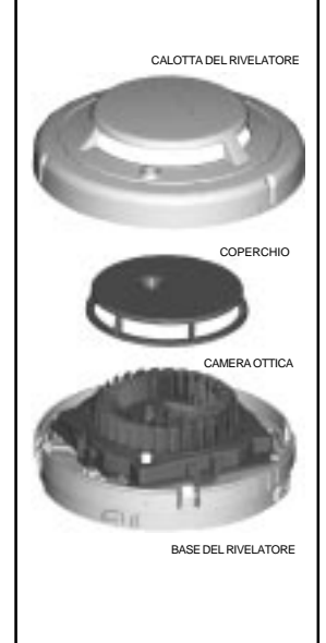
Figura 3: Rivelatore Ottico di Fumo SD-851E
