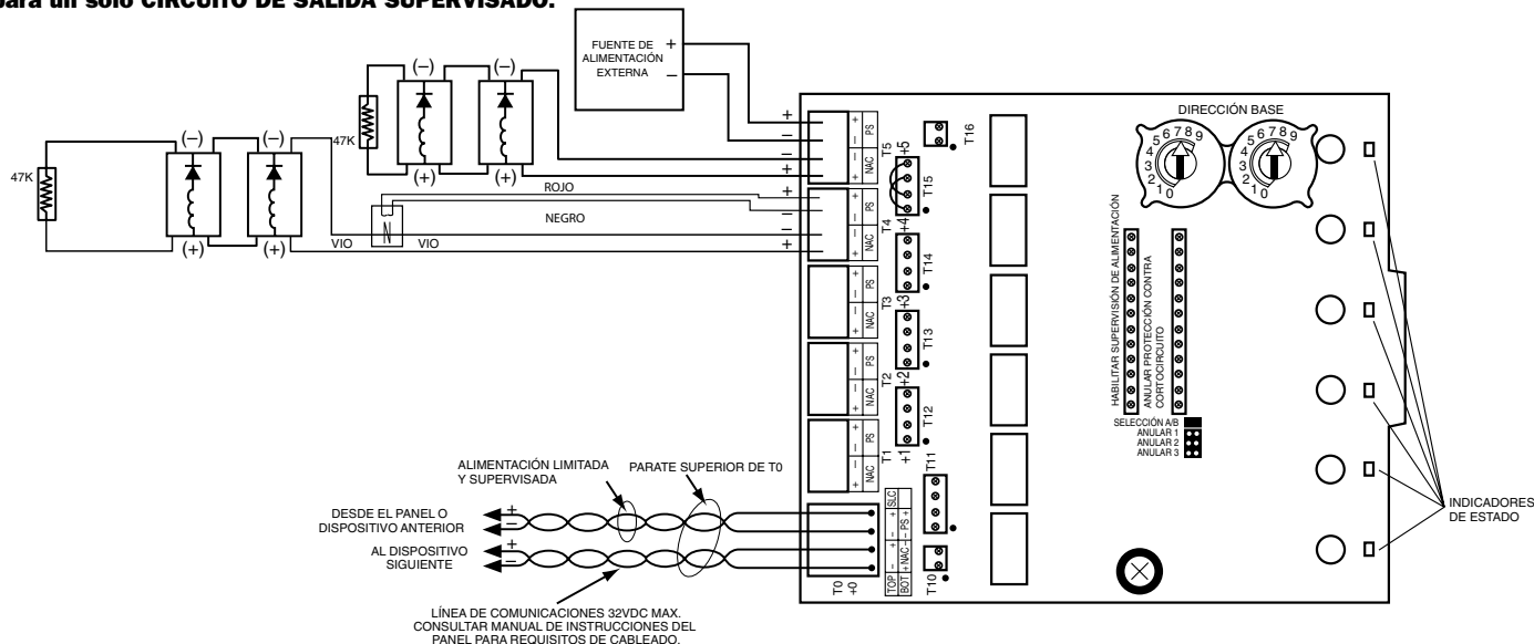
Figura 3: Ejemplo de configuración del CIRCUITO DE SALIDA SUPERVISADO en Clase B, Estilo Y con una única fuente de alimentación compartida por dos CIRCUITOS DE SALIDA SUPERVISADOS.
