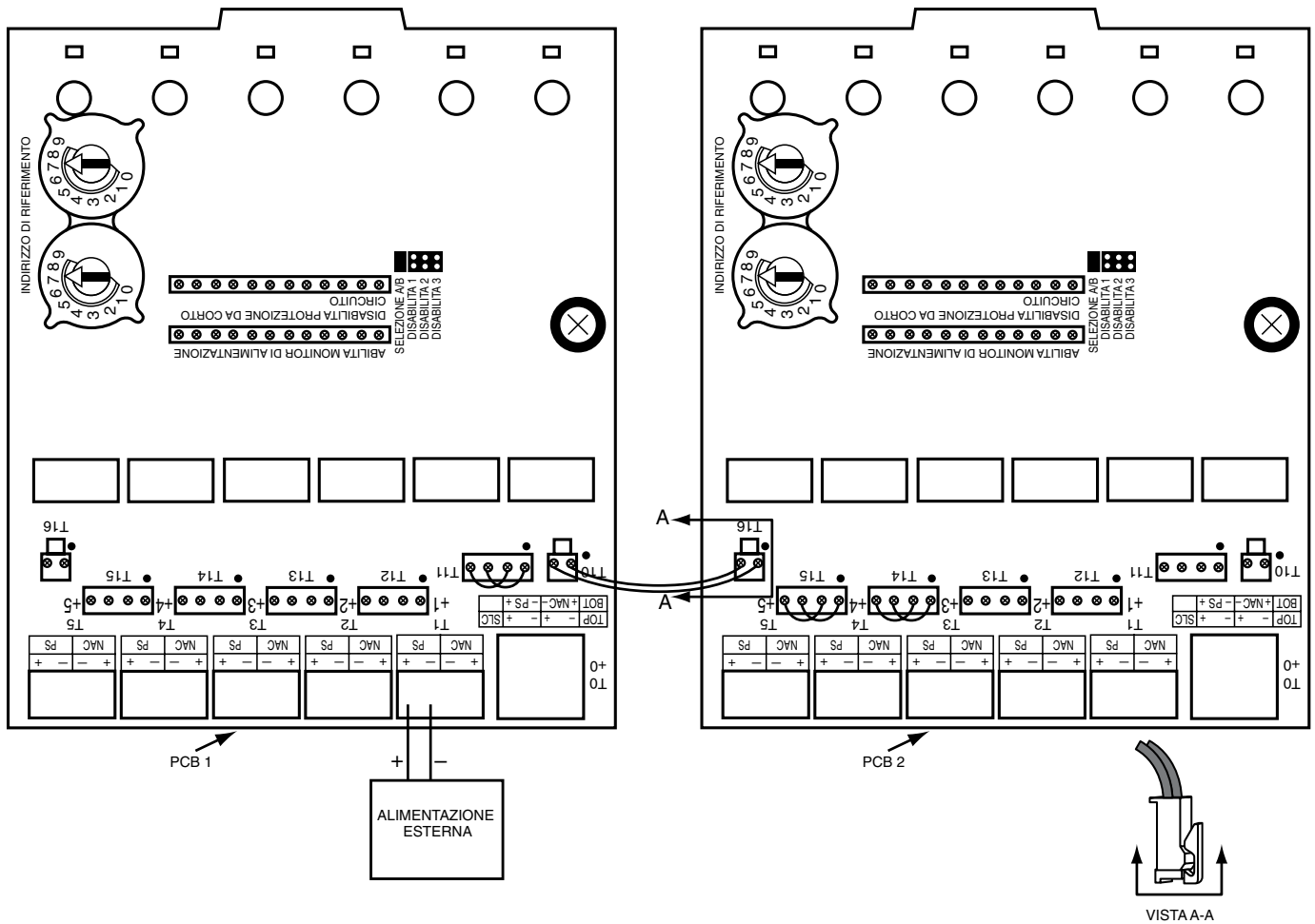
Figura 4: Esempio di più schede che condividono la stessa alimentazione esterna. L'alimentazione è condivisa dai Circuito D'uscita Supervisionato (M.O.C.) +0 e +1 (sulla PCB 1) e da +3, +4 e +5 (sulla PCB 2). Per informazioni sul cablaggio M.O.C. tipico, fare riferimento alle figure 9-12. Verificare che la piegatura del bordo sul jumper di alimentazione lungo si agganci alla linguetta di fissaggio su T10 o T16 come mostrato nella vista A-A.
