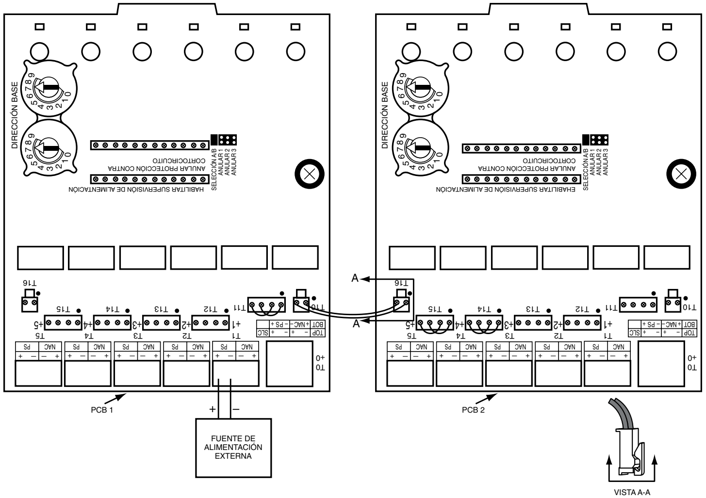
Figura 4: Ejemplo de varias tarjetas que comparten la misma fuente externa de alimentación. La alimentación la comparten los CIRCUITOS DE SALIDA SUPERVISADOS +0 y +1 (de la PCB 1) así como los +3, +4 y +5 (de la PCB 2). Consulte las figuras 3 para ver un ejemplo de cableado típico del CIRCUITO DE SALIDA SUPERVISADO. Asegúrese de que el conector del puente de alimentación largo encaja correctamente en la pestaña de sujeción en T10 o T16, como se muestra en Vista A-A.
