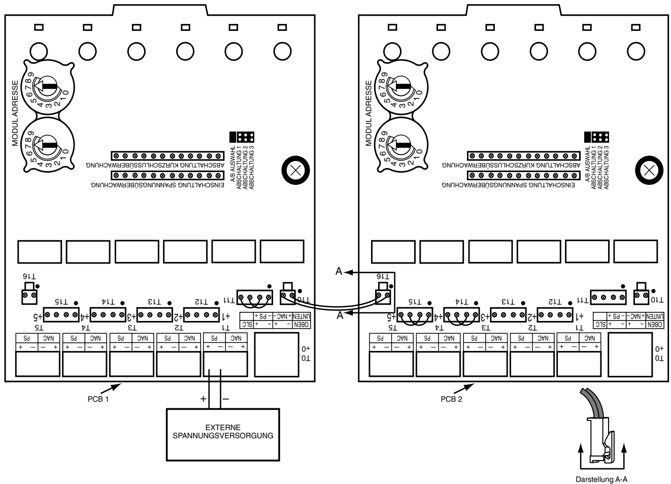
Abbildung 4: Beispiel zur gemeinsamen Spannungsversorgung von Modulen. Die Versorgungsspannung wird auch zur Versorgung der überwachten Steuerausgänge +0 and +1 (auf Platine 1) sowie +3, +4, and +5 (auf Platine 2) genutzt. Die Abbildungen 3 zeigen die typische Verdrahtung der Ausgangskreise. Vergewissern Sie sich dass der Stecker des Spannungskabel, wie in der Darstellung A-A gezeigt, fest in den Halteclip von T10 oder T16 einrastet.
