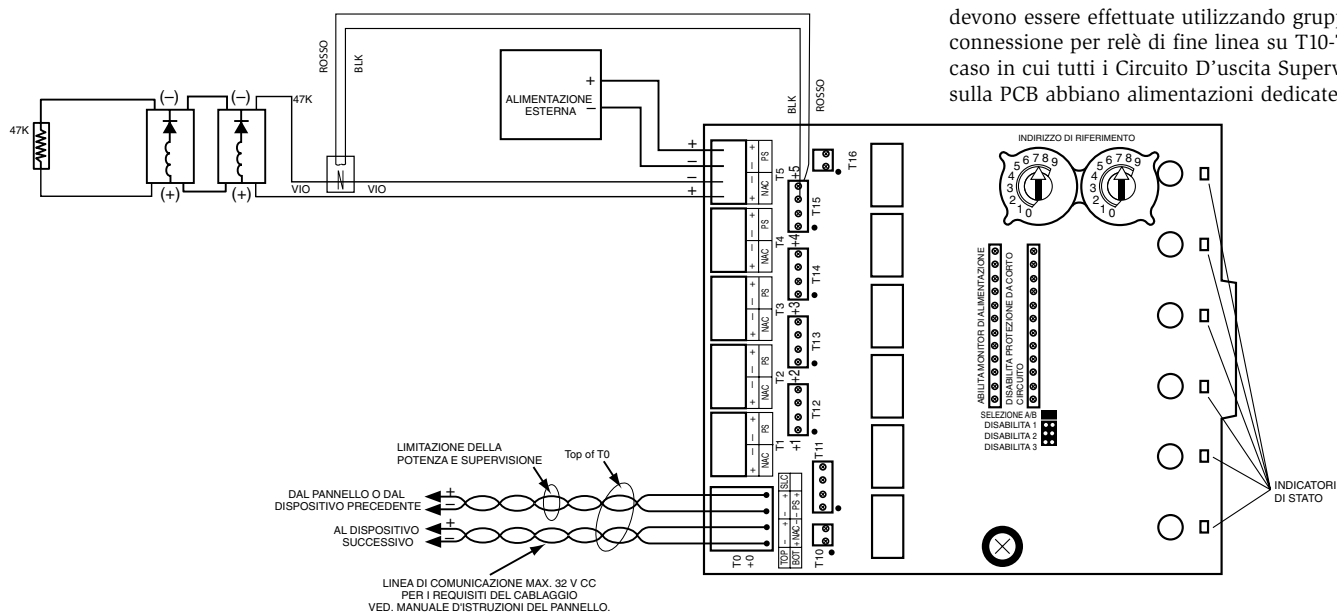
Figura 2: Esempio di configurazione Circuito D'uscita Supervisionato Classe B, tipo Y con una singola alimentazione dedicata ad un singolo Circuito D'uscita Supervisionato.
