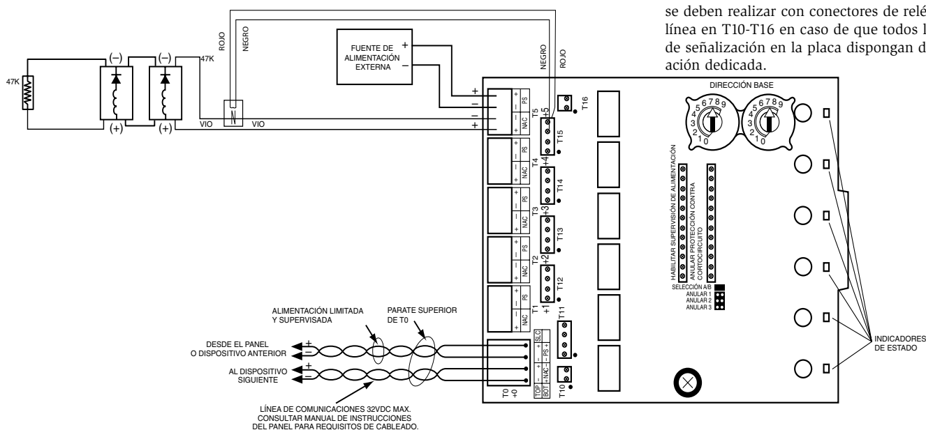
Figura 2: Ejemplo de configuración del CIRCUITO DE SALIDA SUPERVISADO en Clase B, Estilo Y con una única fuente de alimentación para un sólo CIRCUITO DE SALIDA SUPERVISADO.
