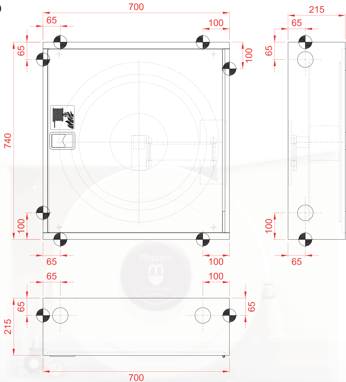
DIMENSIONES EMPOTRAMIENTO
