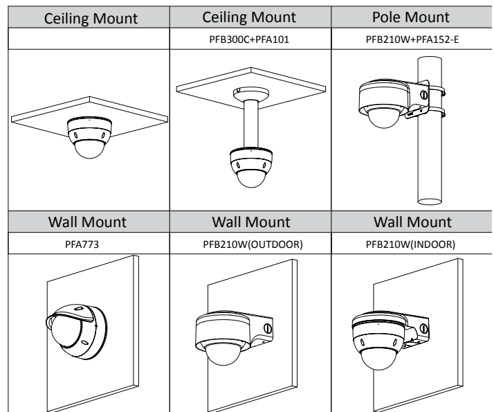
PFA773 Wall Mount
